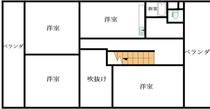
二階平面図
